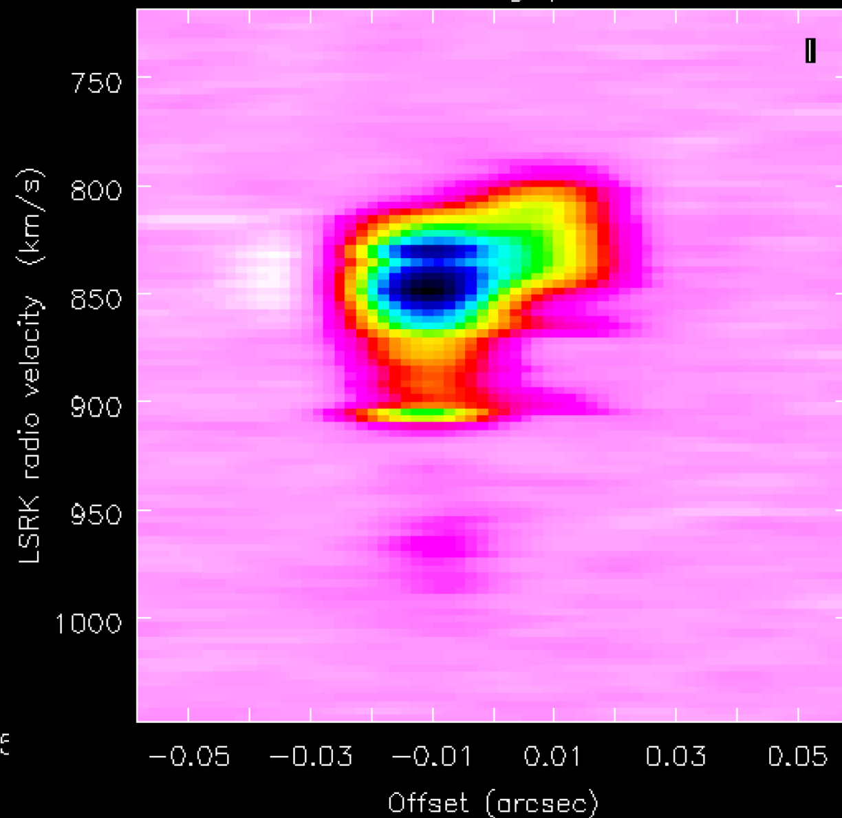
NGC660_line.clean.image.pvline.001-raster
