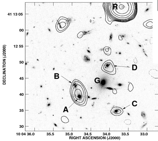
New global VLBI (Zhang et al.)
